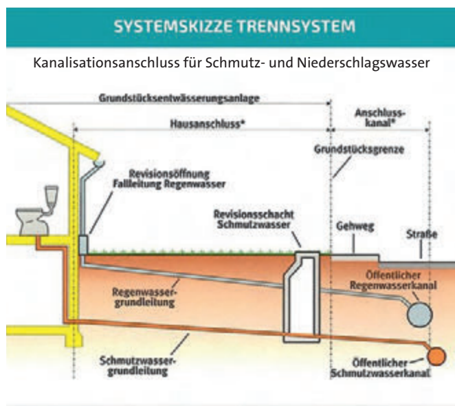
Grundstücksanschluss: öffentlicher und privater Bereich
