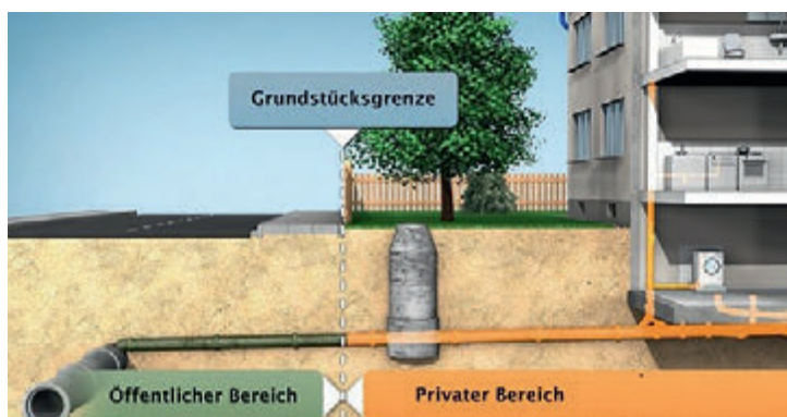
Grundstücksanschluss: öffentlicher und privater Bereich
